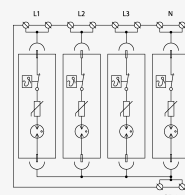
Schéma zapojení
